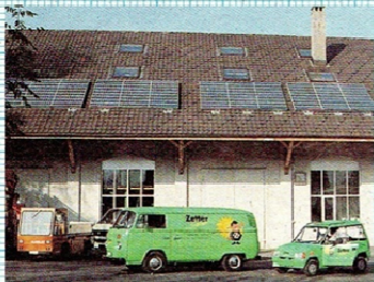
9-kW-Solarzellenanlage Olten
