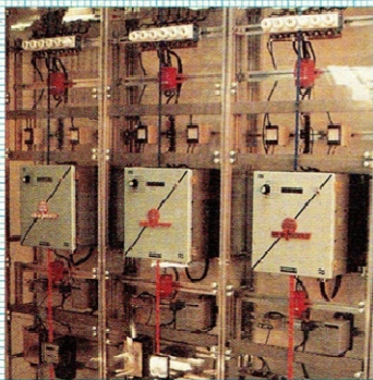
El.-Tableau (Wechselrichter 3x SI-3000)
